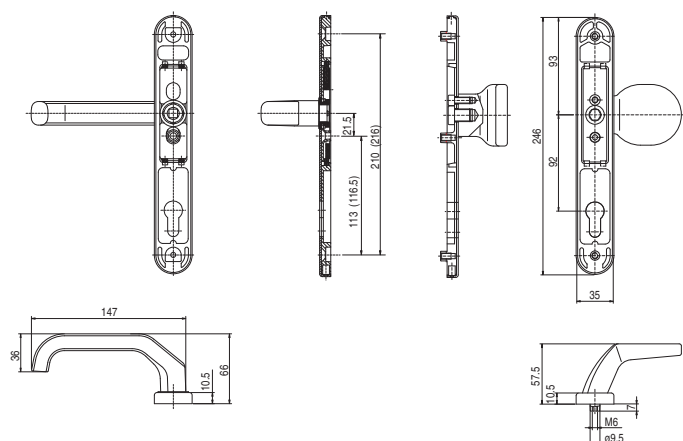
Klamka drzwiowa z pochwytem
