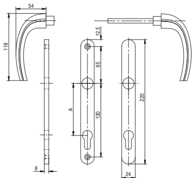
Klamka drzwiowa ze śrubą imbusową M6
