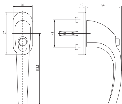
Klamka okienna z przyciskiem
