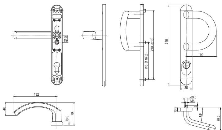
Klamka drzwiowa z pochwytem P
