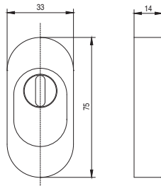
Szyld wkładki patentowej z antywłamaniową ochroną
