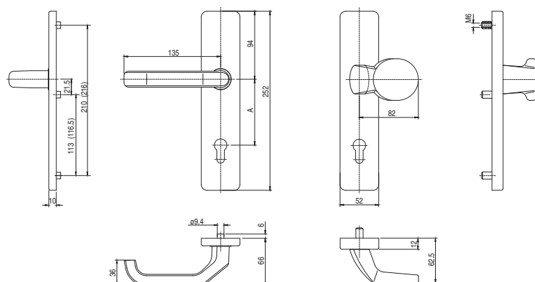
Klamka drzwiowa z gałką
