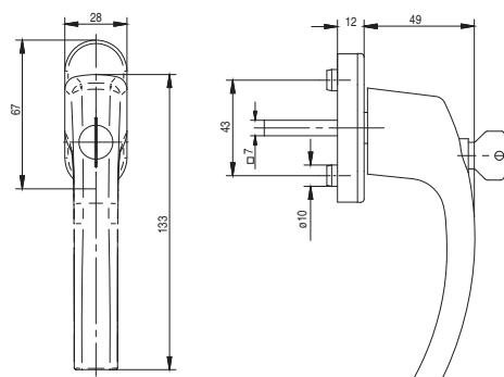
Klamka okienna z kluczykiem z funkcją TBT (Tilt Before Turn)
