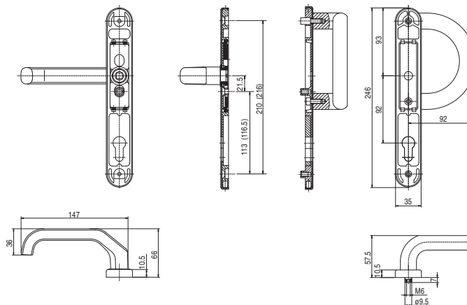
Klamka drzwiowa z pochwytem
