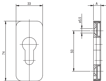
Szyld wkładki patentowej prostokątny
