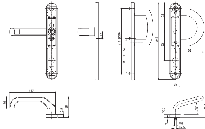
Klamka drzwiowa z pochwytym typu P
