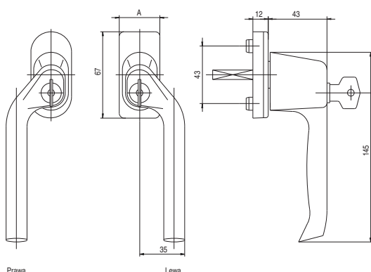
Klamki okienne do okien otwieranych na zewnątrz
