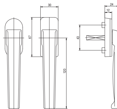
Klamka okienna pod żaluzję
