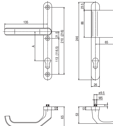
Klamka drzwiowa z pochwytem typu L
