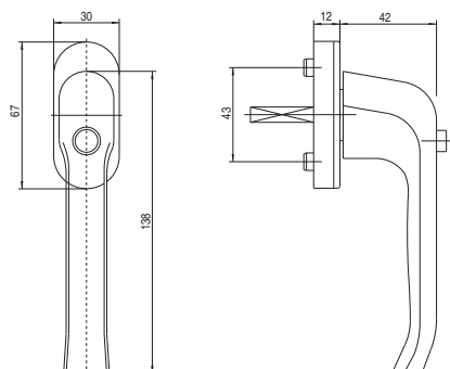
Klamka okienna z przyciskiem
