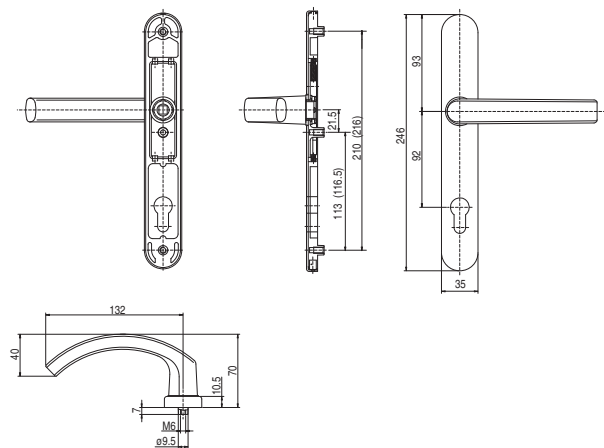
Klamka drzwiowa z gałką
