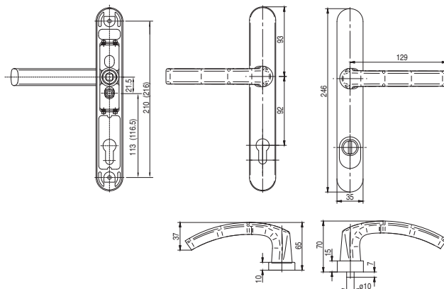
Klamka drzwiowa
