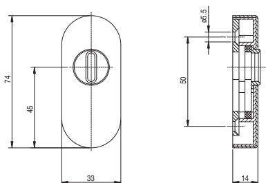
Szyld wkładki patentowej z antywłamaniową ochroną
