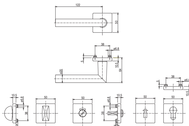
Klamka drzwiowa wewnętrzna
