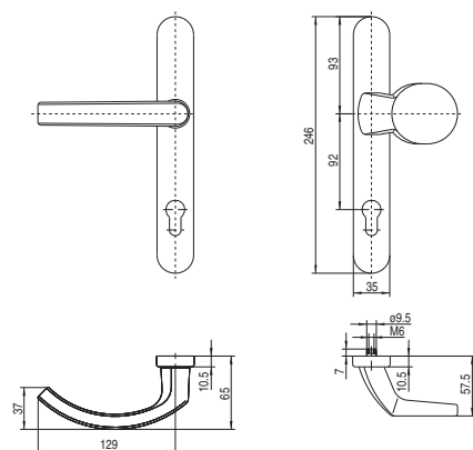
Klamka drzwiowa z pochwytem typu P
