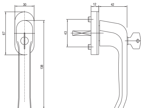
Klamka okienna z kluczykiem
