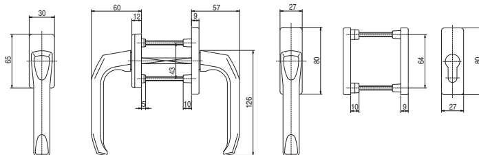
Komplet balkonowy
