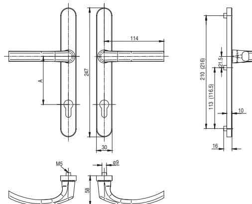
Klamka drzwiowa z pochwytem typu L
