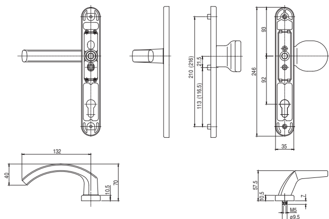
Klamka drzwiowa z pochwytem V
