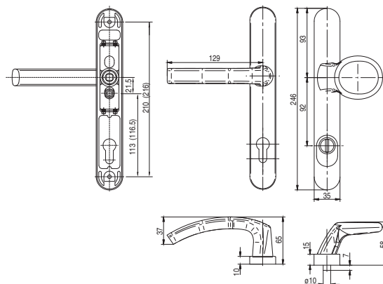
Klamka drzwiowa z gałką
