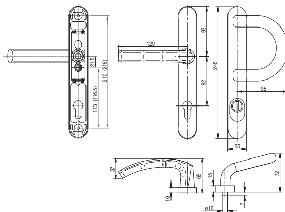
Klamka drzwiowa z pochwytem P
