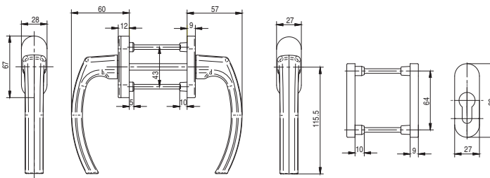
Komplet balkonowy z szyldami owalnymi
