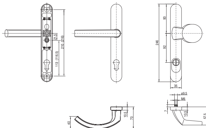
Klamka drzwiowa z gałką
