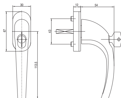
Klamka okienna z kluczykiem
