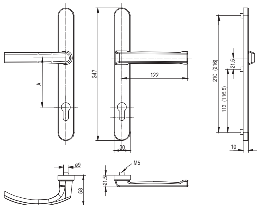
Klamka drzwiowa pod żaluzję
