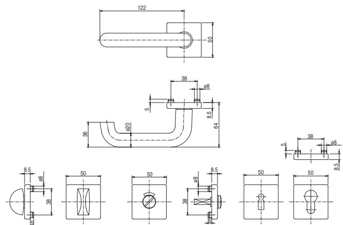
Klamka drzwiowa wewnętrzna
