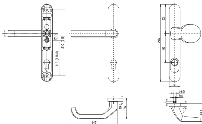
Klamka drzwiowa z gałką
