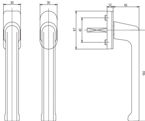
Klamka do drzwi przesuwnych z kluczykiem
