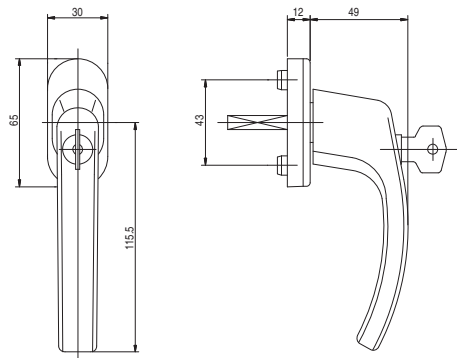
Klamka okienna antywłamaniowa
