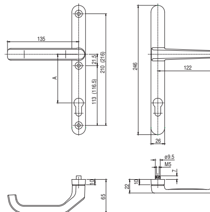
Klamka drzwiowa z pochwytem typu L
