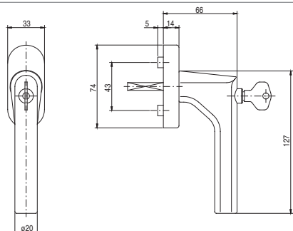
Klamka okienna z kluczykiem
