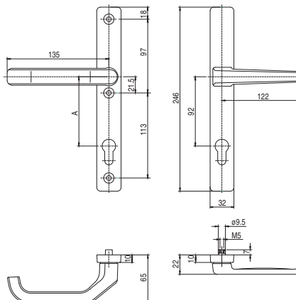
Klamka drzwiowa z pochwytem typu L
