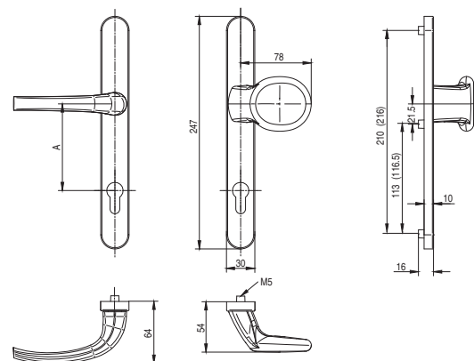
Klamka drzwiowa z gałką
