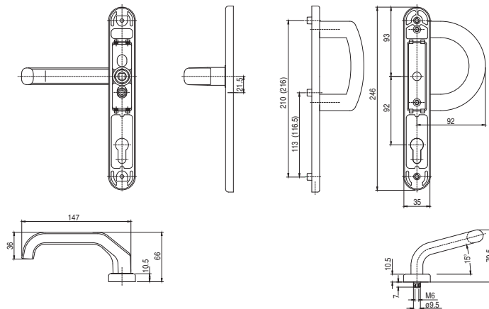
Klamka drzwiowa z pochwytem typu P
