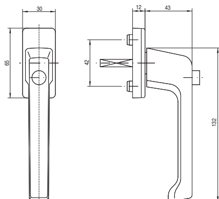
Klamka okienna z przyciskiem
