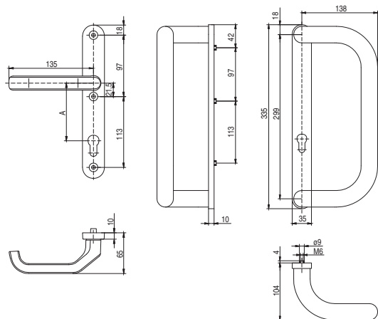
Klamka drzwiowa z pochwytem prostokątnym
