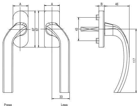
Klamki okienne do okien otwieranych na zewnątrz
