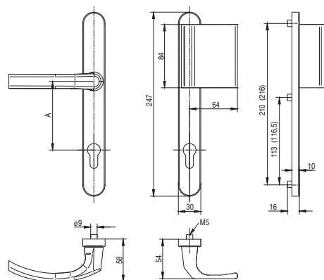
Klamka drzwiowa z pochwytem typu L
