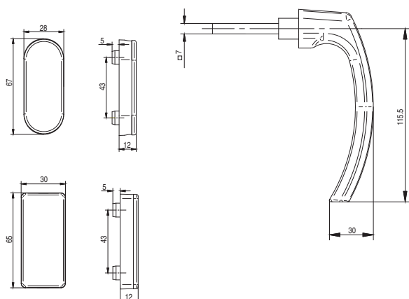
Klamka okienna z rozetą ślepą prostokątną i owalną
