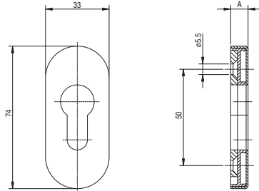
Szyld wkładki patentowej owalny
