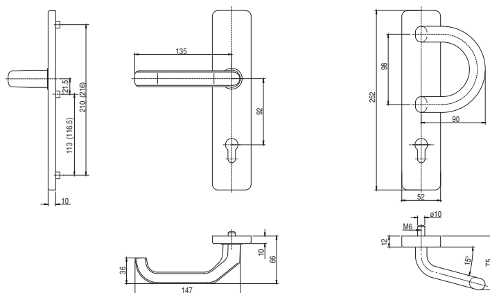
Klamka drzwiowa z pochwytem typu P
