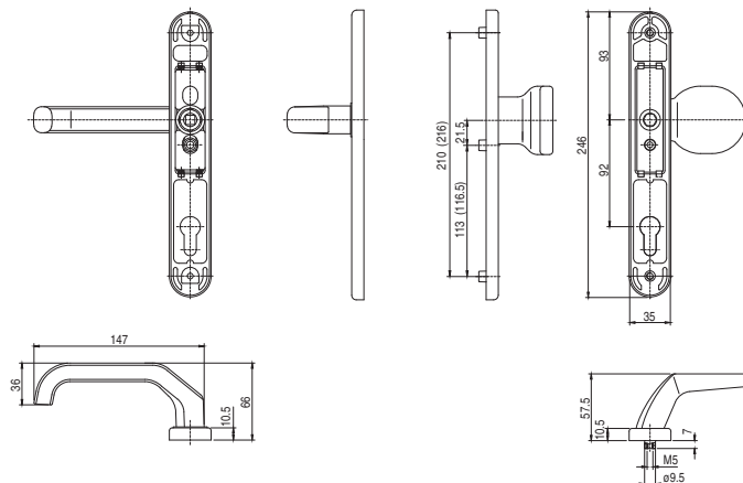
Klamka drzwiowa z pochwytym typu P
