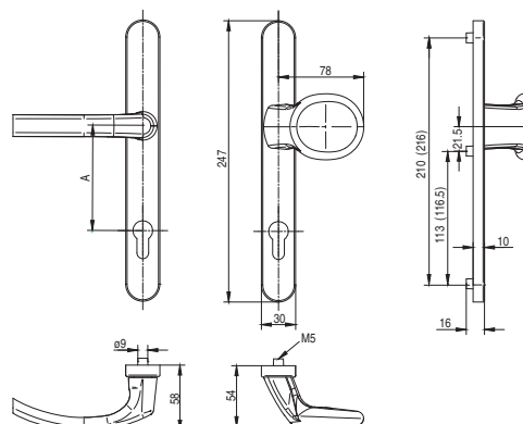
Klamka drzwiowa z gałką
