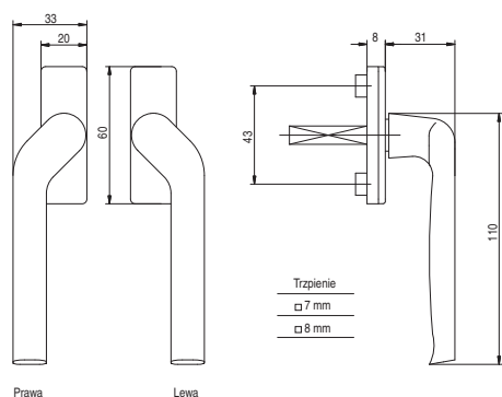
Klamki okienne do okien otwieranych na zewnątrz średnica czopów tylko 10mm
