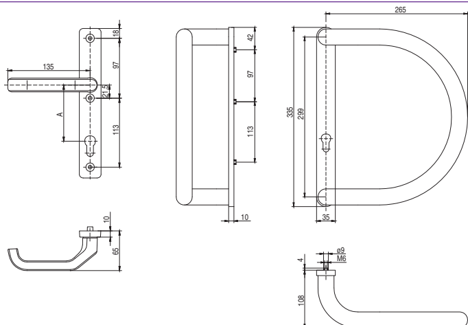
Klamka drzwiowa z pochwytem półokrągłym
