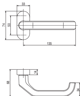
Klamka drzwiowa dzielona z szyldem owalnym
