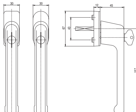
Klamka do drzwi przesuwnych z kluczykiem
