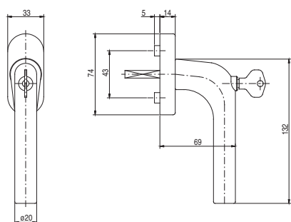
Klamka okienna z kluczykiem
