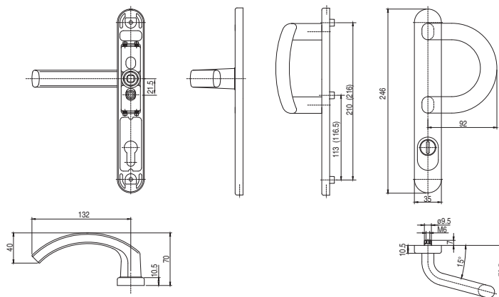
Klamka drzwiowa z pochwycem typu P
