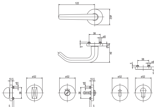
Klamka drzwiowa wewnętrzna
